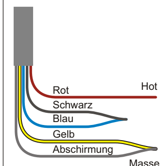
Pickup-Kabel
