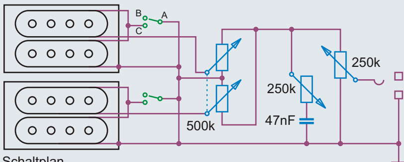
Schaltplan
