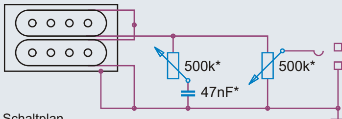
Schaltplan
